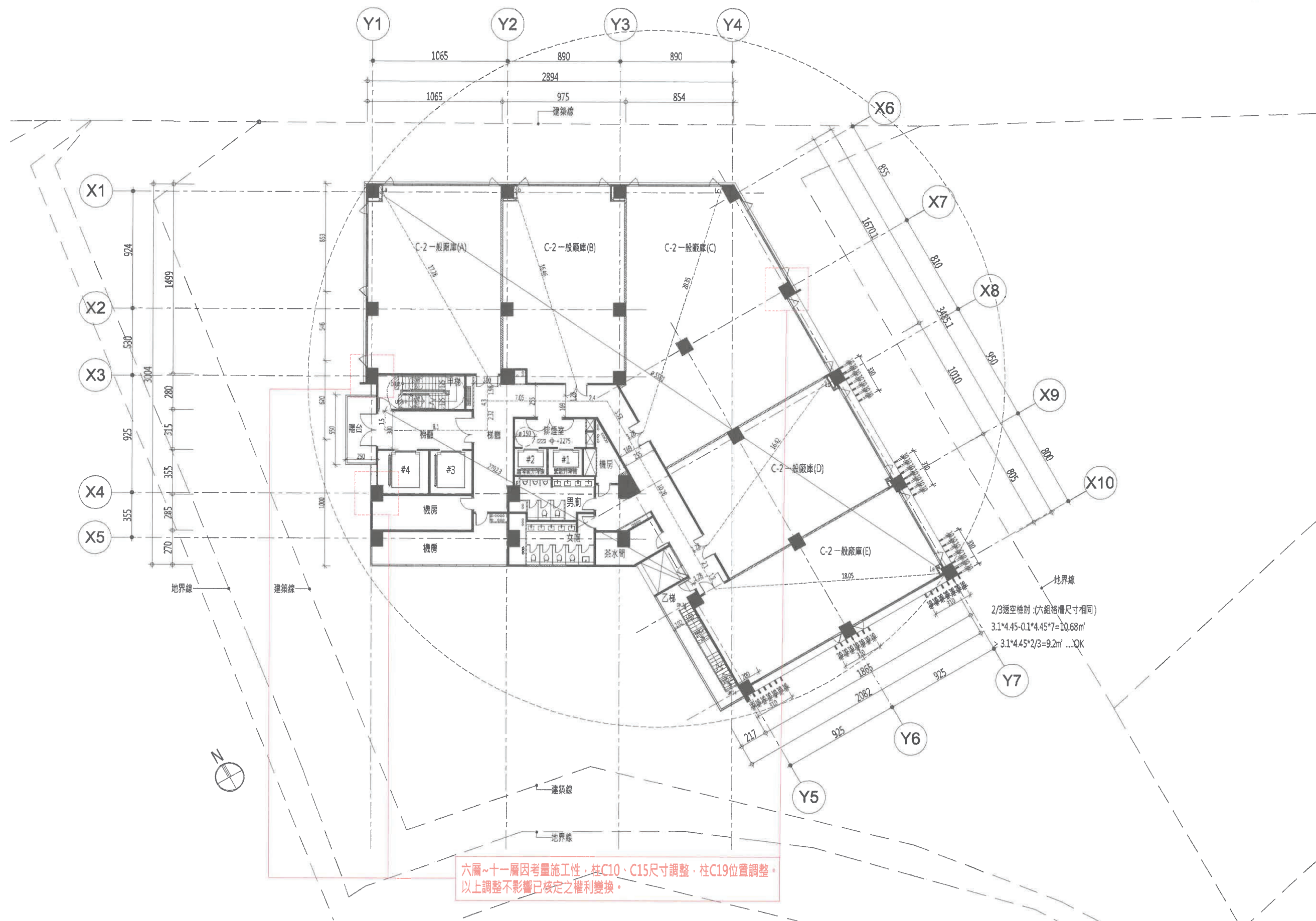
圖 6-11-1 地上六層平面圖(S : 1/300)
