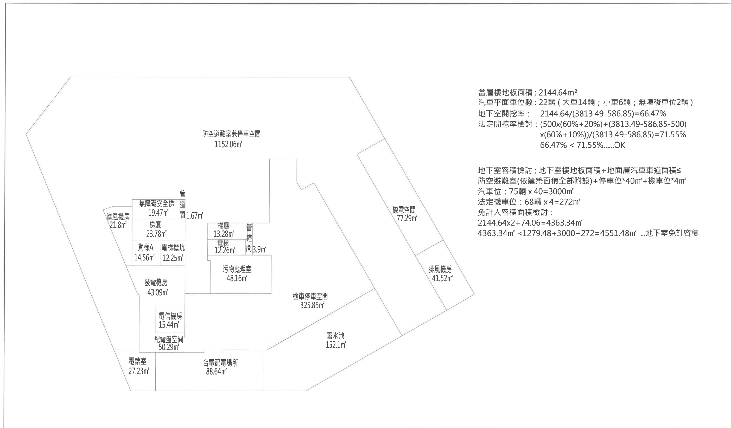
圖 6-26 地下一層面積檢討圖(S：1/300)
