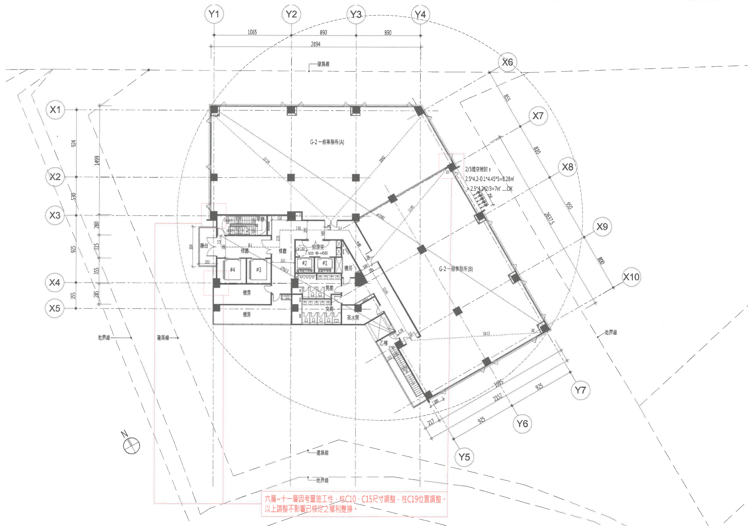
圖 6-21-1 地上十一層平面圖(S : 1/300)
