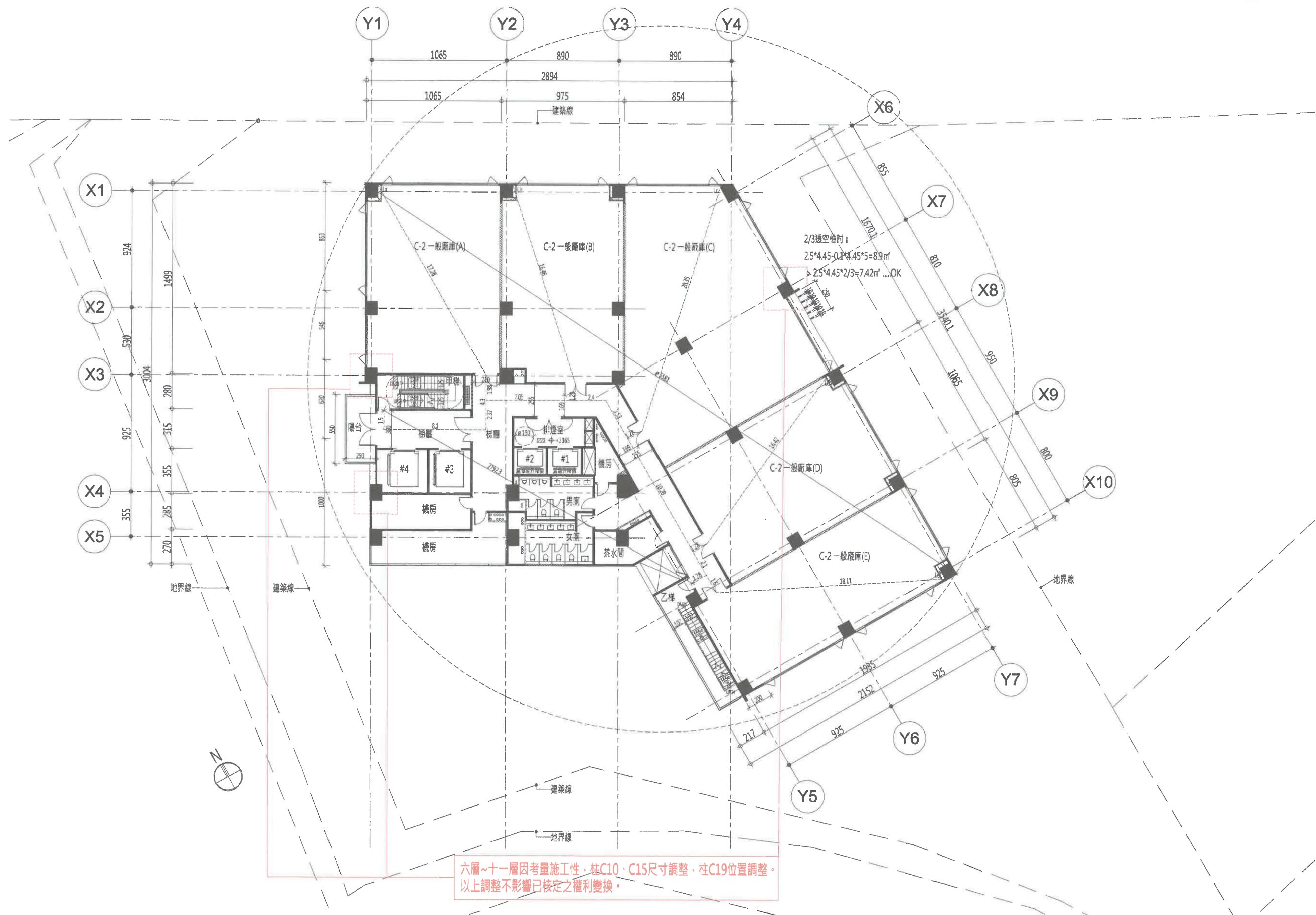
圖 6-15-1 地上八層平面圖(S : 1/300)
