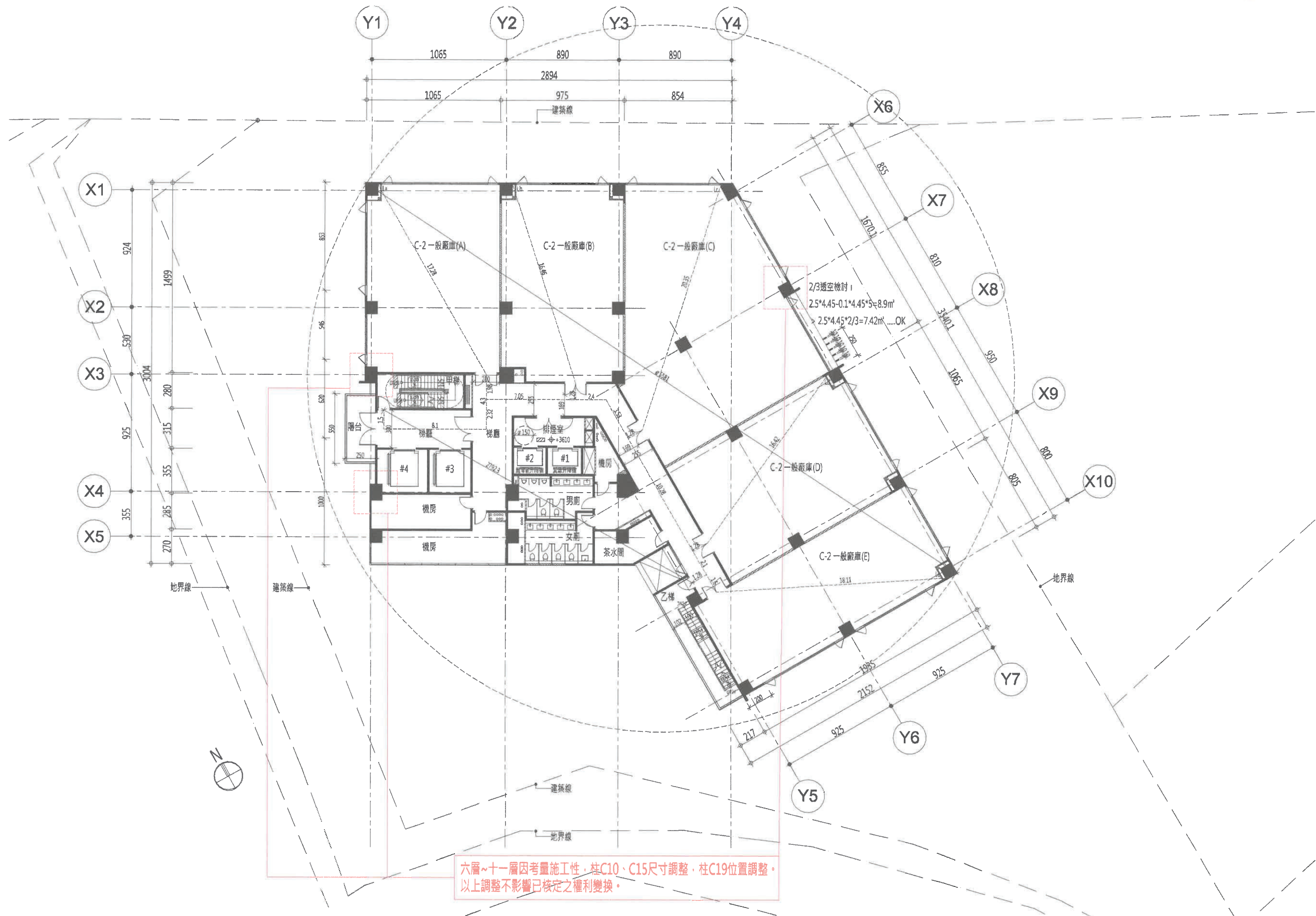
圖 6-17-1 地上九層平面圖(S : 1/300)
