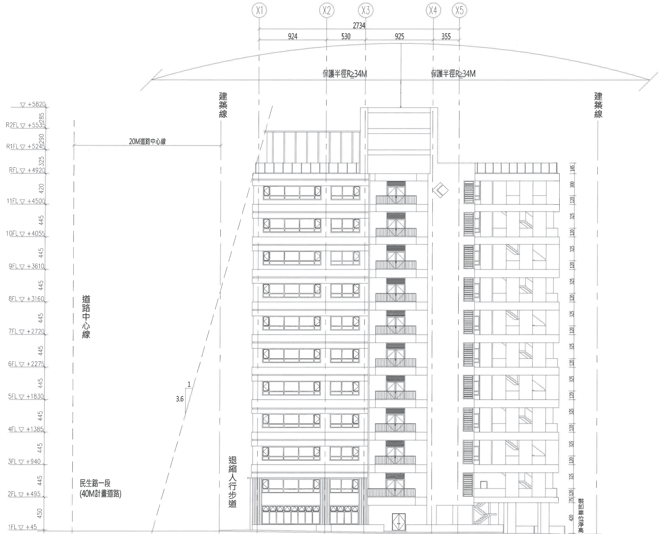
圖 6-34 西北向立面圖(S : 1/300)
