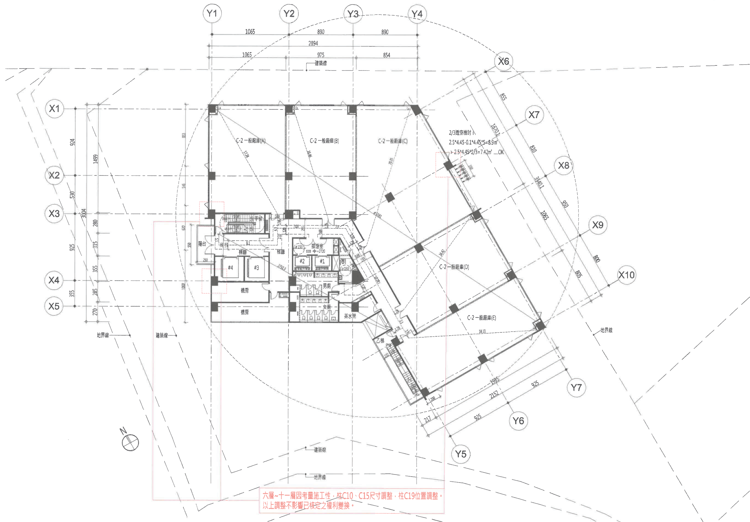
圖 6-13-1 地上七層平面圖(S : 1/300)
