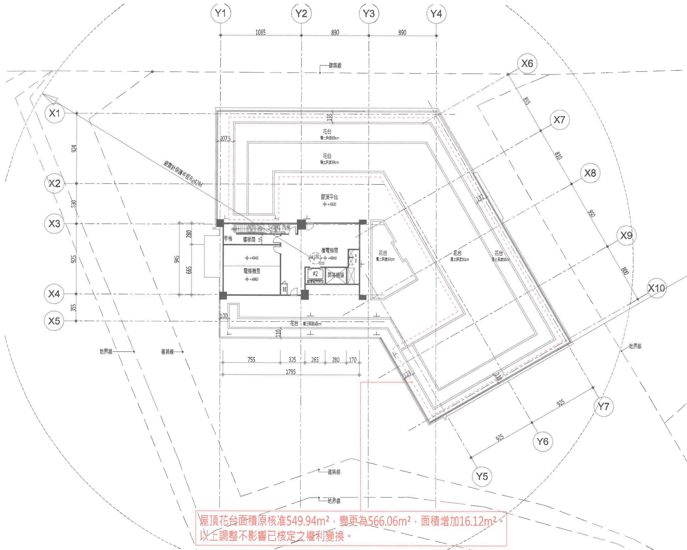
圖 6-23-1 屋突層平面圖(S : 1/300)
