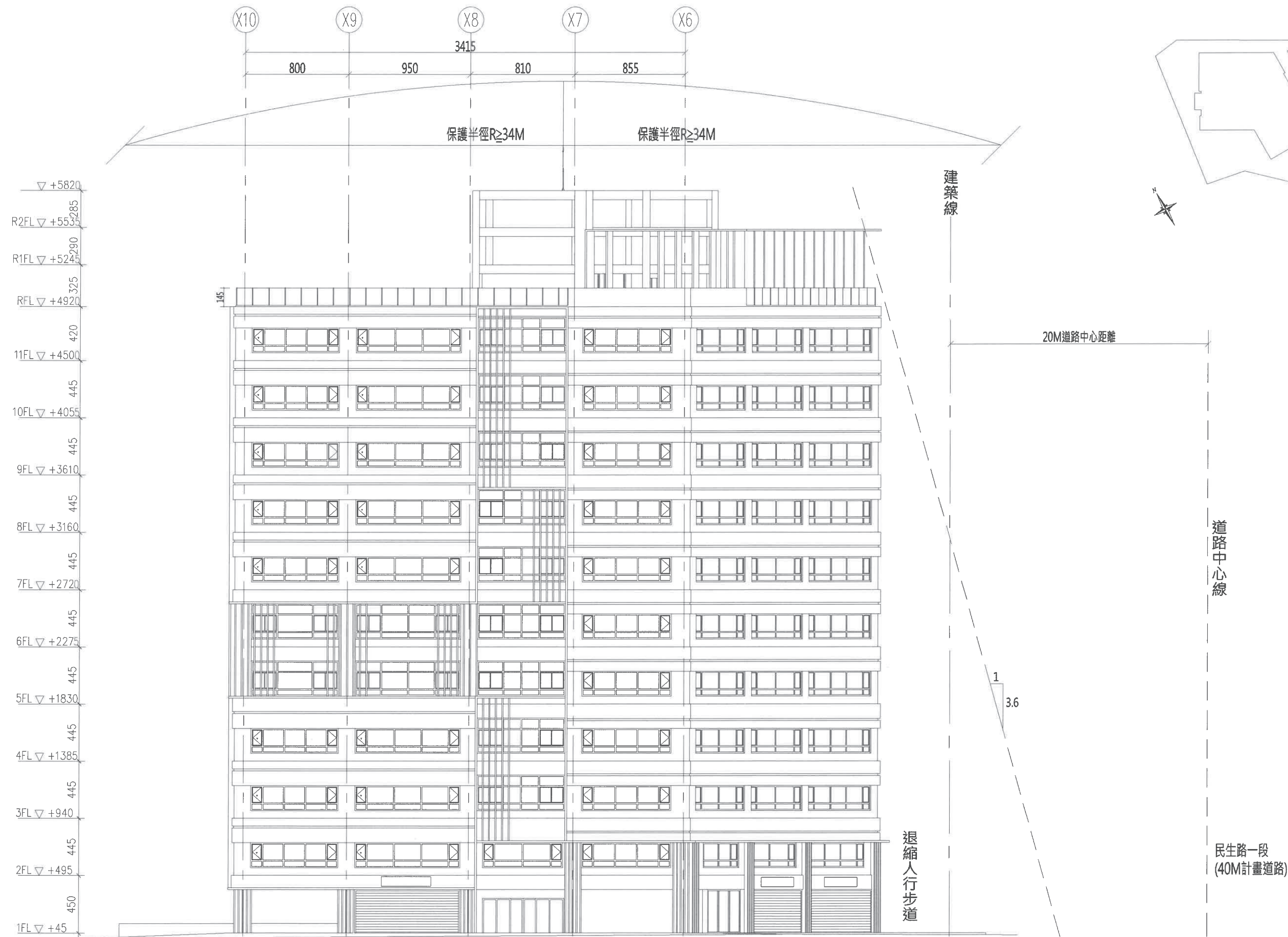
圖 6-30 東向立面圖(S : 1/300)
