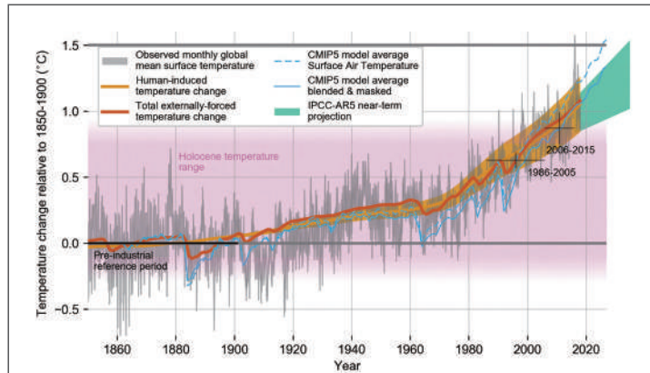
全球平均地表溫度演變 圖片來源： https://www.ipcc.ch/sr15/graphics/
